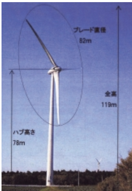
風車外形図
