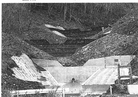
▼整備された天田沢
