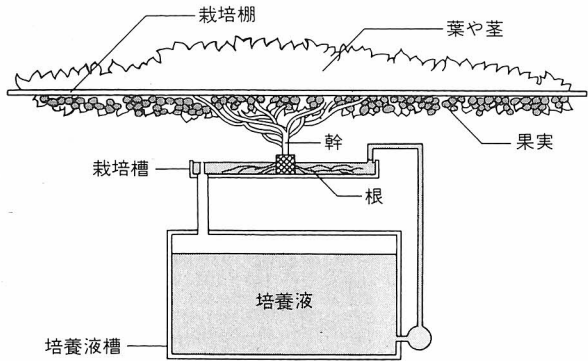
水気耕栽培装置のシステム / Hydroponics System
