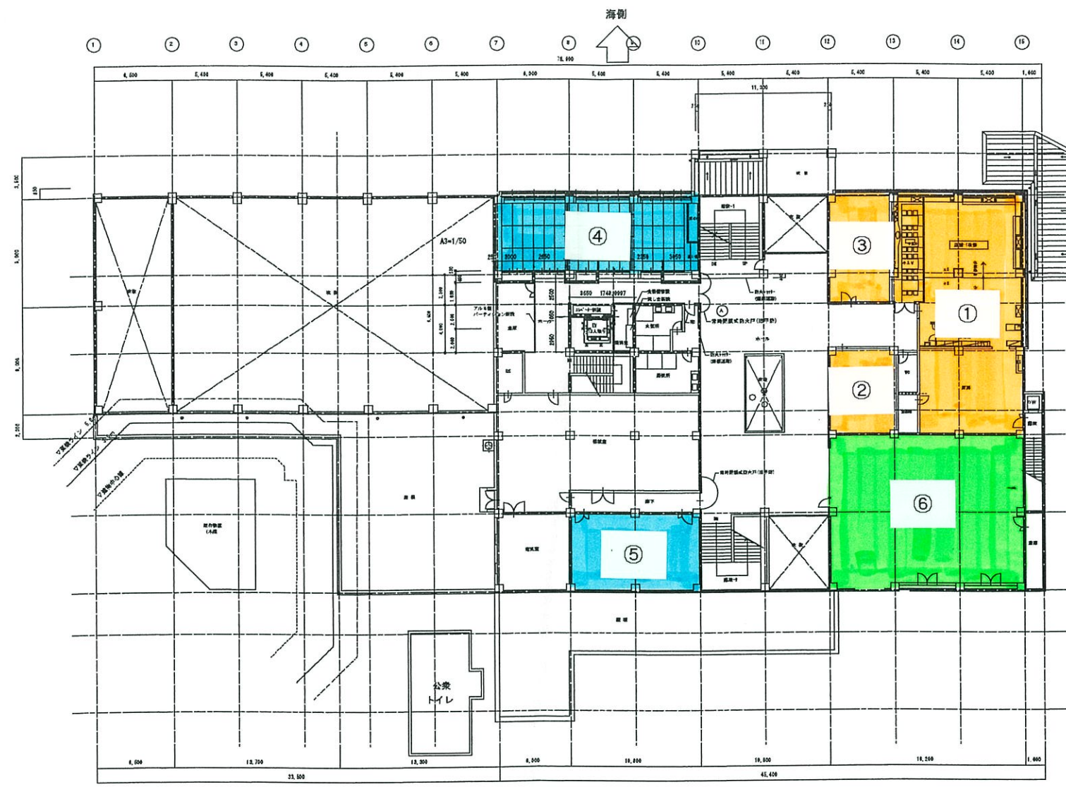
改修後 2階平面図 1/200
